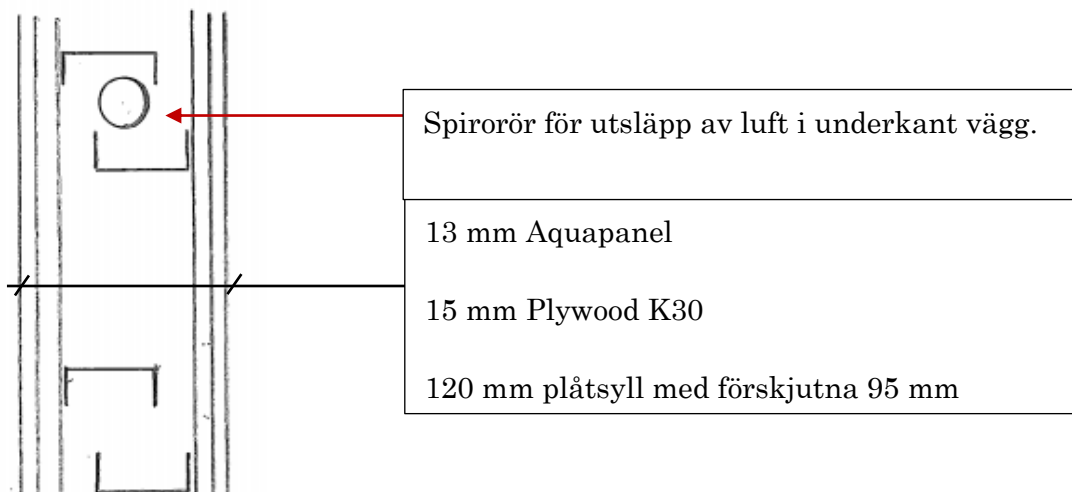
Bild 3 – Principskiss över utförande av ventilerad väggstomme som kan belastas med tvåsidig vattenbelastning
