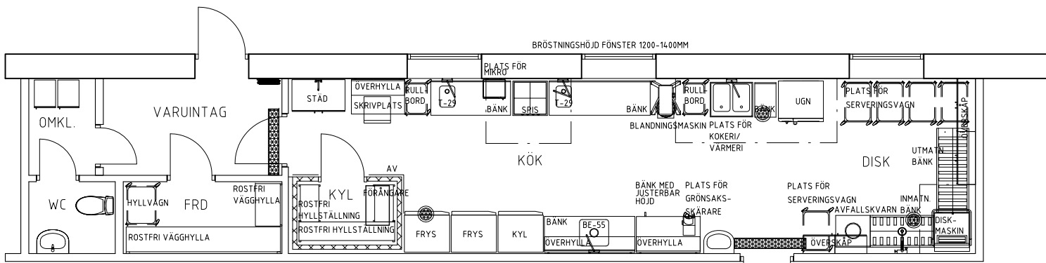
EXEMPEL PLANLÖSNING AVLÅNGT KÖK, 4 AVD.
