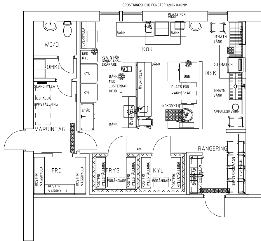
EXEMPEL PLANLÖSNING KVADRATISKT KÖK 6 AVD
