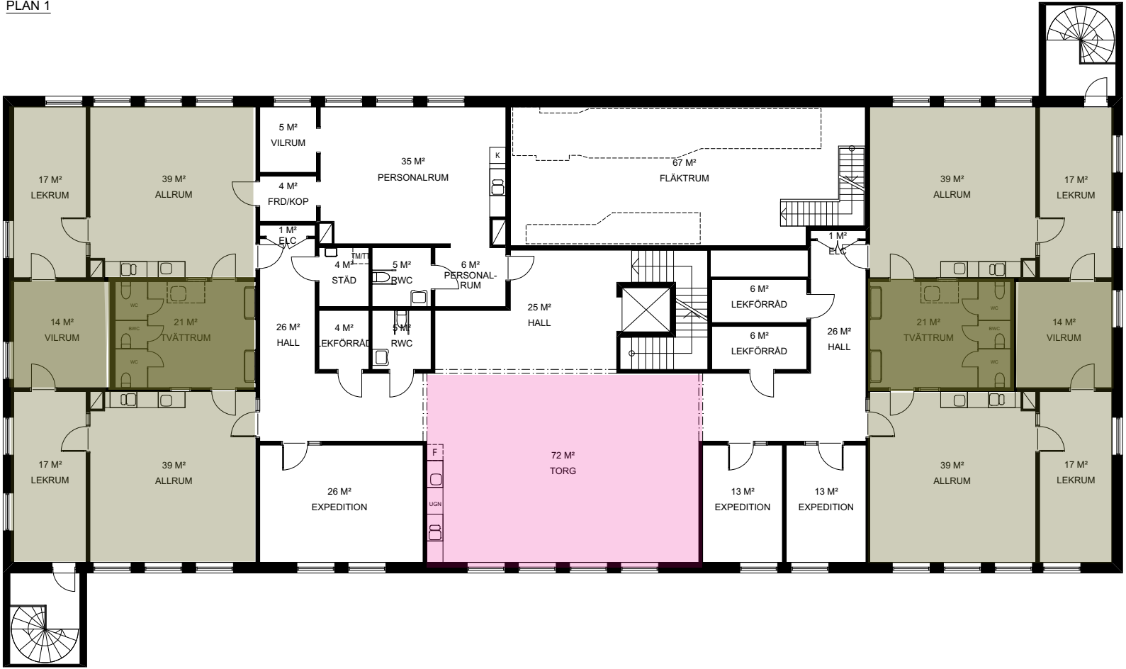
Övre plan
