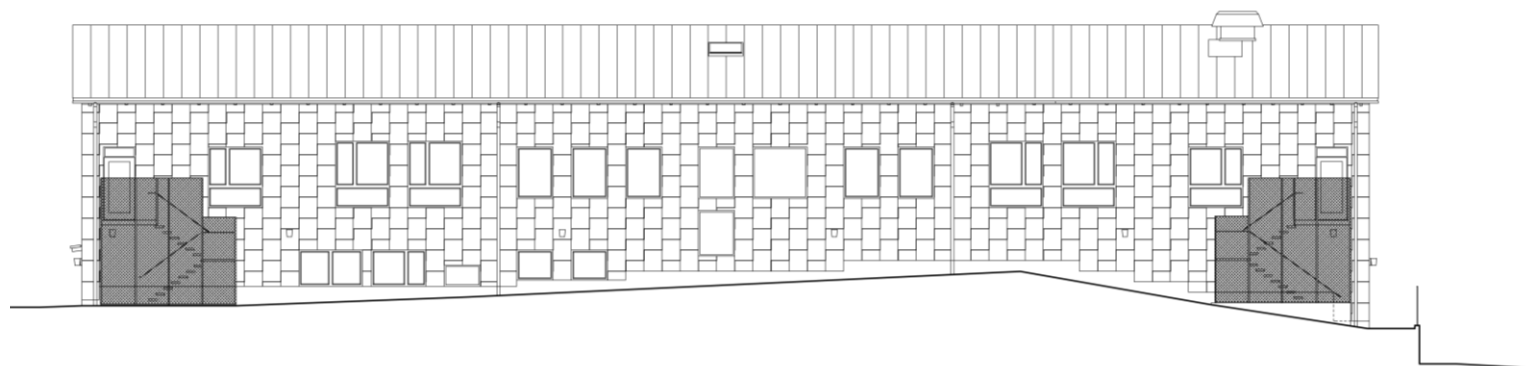
FASAD MOT SYDÖST
