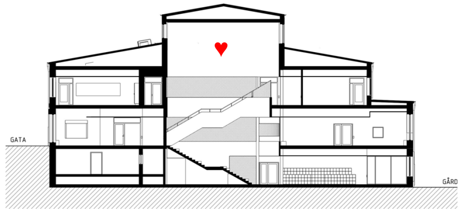
Sektion A-A
